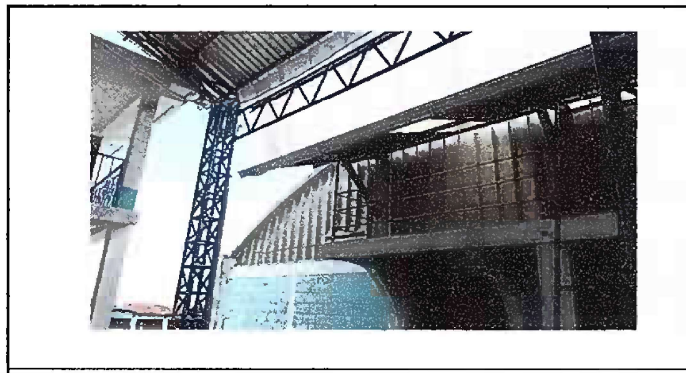
Foto No. 11 MODULO 5 Sustitución de bajada de agua pluvial de tubo PVC 3 y sustitución de canales PVC.
