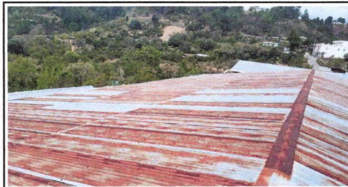
Foto 3: Módulo 1. Sustitución de lámina por lámina troquelada aluzinc cal. 26
