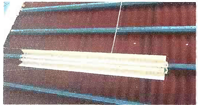
Foto 4: Sustitucion de plafoneras, cajas octogonales y bombillas
