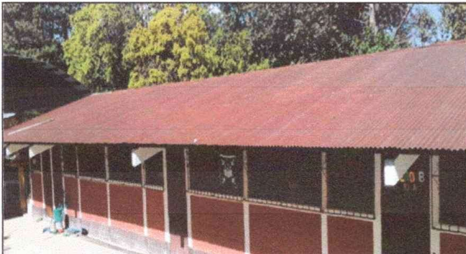
FOTO 3 MODULO 1: Sustitución de elementos de fijación (Tornillos) en techado.
