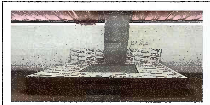
Foto 5: (MODULO 2). Se ha terminado la colocación de azulejos en las respectivas planchas de la cocina del establecimiento
