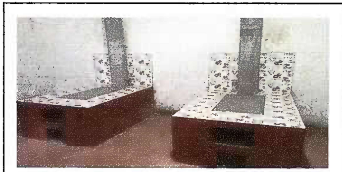
Foto 6: (MODULO 2). Las dos planchas fueron terminadas exitosamente en la escuela.
