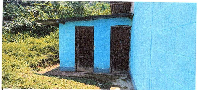
Foto 4: MODULO 2, Sustitución de laminas, por laminas troqueladas aluzinc calibre 26
