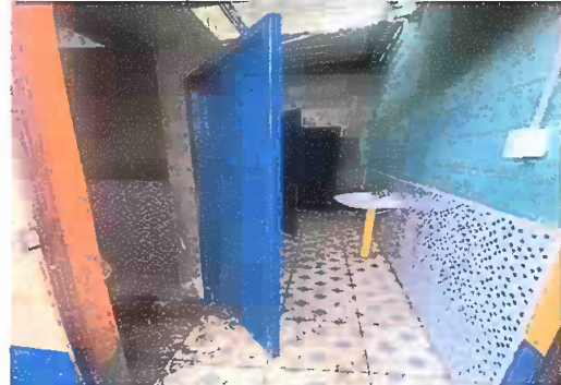
Foto 6. MODULO 3: Suministro e Instalación de puertas de metal en sanitarios
