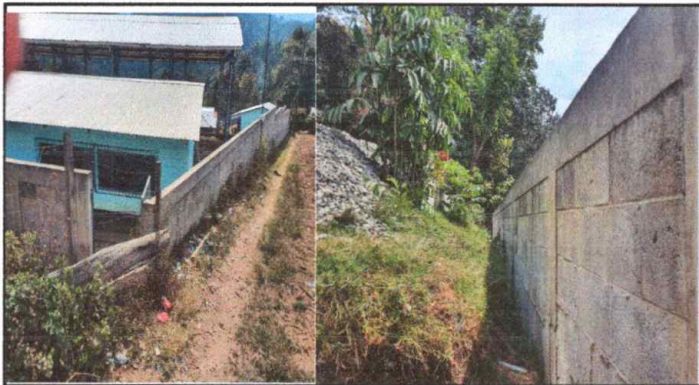
Foto 3: Reparación de muro perimetral de block con tubo hg y malla galvanizada para la seguridad del establecimiento, por la altura de la pared.
