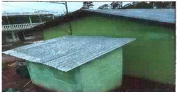
Foto 6: MODULO 2, sustitución de lámina, por lámina troquelada aluzcinc calibre 26
