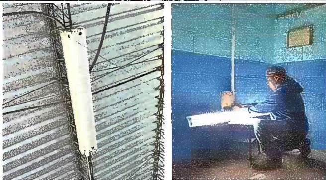
FOTO 15. MÓDULO 4: Sustitución de lámparas 2 x 40
