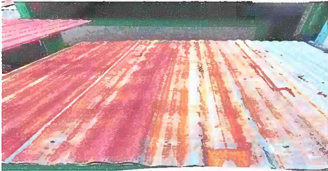
Foto 7: Modulo 2 Sustitución de lámina por lámina troquelada aluzinc calibre 26, Instalación de lámina troquelada aluzinc, Sustitución de elementos de fijación (tornillos).
