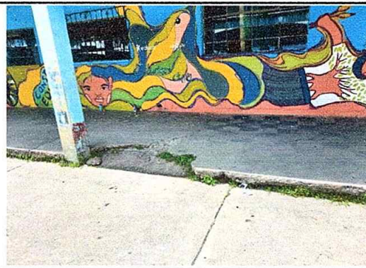
Foto 4: Reparación de banquetas de concreto, módulo No. 1
