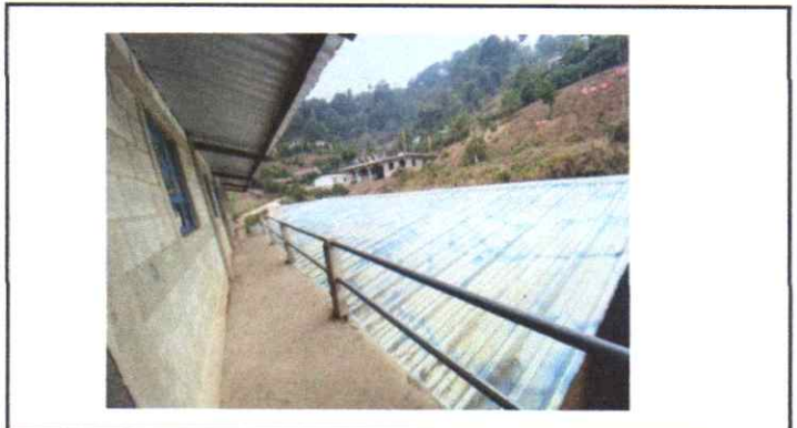
Sustitución de lámina, por lámina troquelada Calibre 26 de 0.40
