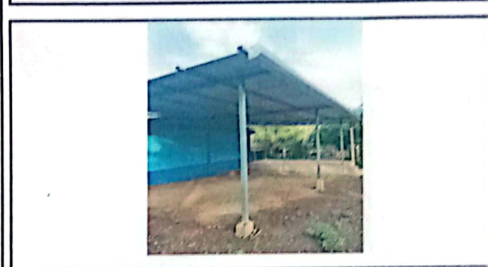
Foto 3: SUSTITUCION E INSTALACION DE LAMINA ALUZINC TROQUELADA C28 EN SALON
