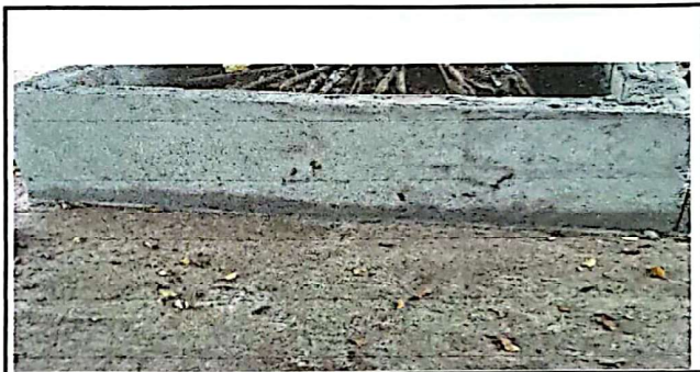
Foto 4: REPARACIÓN DE BORDILLO JARDINERA 1.00X1.00M
