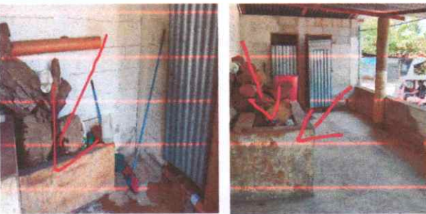
Suministro e instalación de lavamanos de concreto
