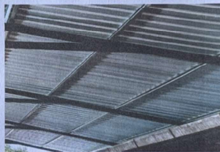
Foto 4: Suministro y sustitución de lámina acanalada por lámina troquelada calibre 26"
