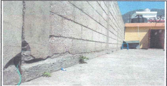
Foto 2: Muro dañado en la base, área donde realizará la reparación con block, columna y solera
