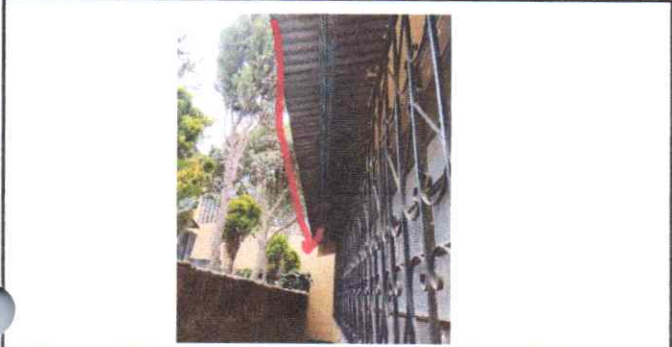
SUSTITUCION DE CANAL T/AMERICANO CALIBRE 28 0.54 X 6.0 M PATIO 2
