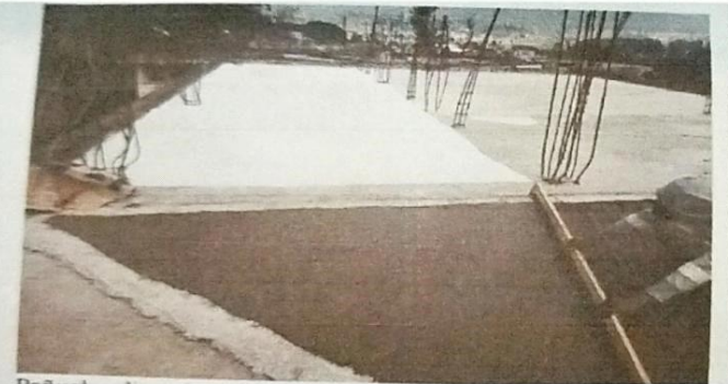
Foto 3: Pañuelos direccionados para bajada de agua pluvial.
