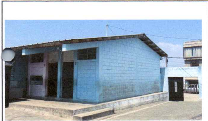
Suministro e instalación de canal con bajada de agua, y suministro e instalación de techo a dos aguas en puerta de ingreso de escuela
