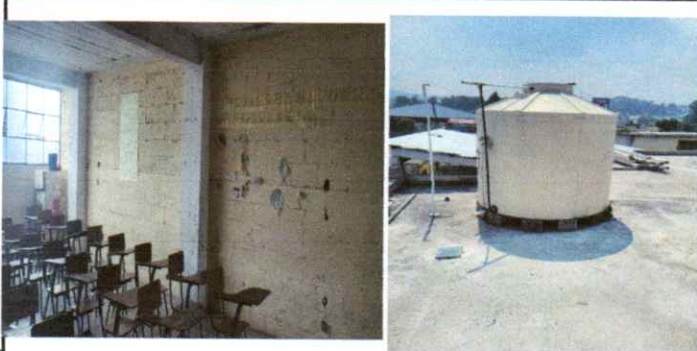
Reparación de muros con repello , Reparación de deposito de agua (2500lt)
