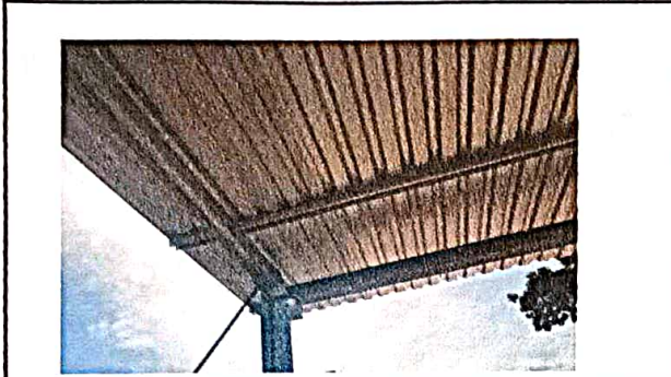
Foto 7: sustitución de lamina por lamina troquelada aluzinc calibre 26 para esenario
