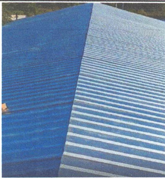
FOTO 3: Sustitución de capote de lámina troquelada
