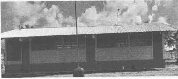
Foto 7: Instalación de lámina troquelada aluzinc calibre 26
