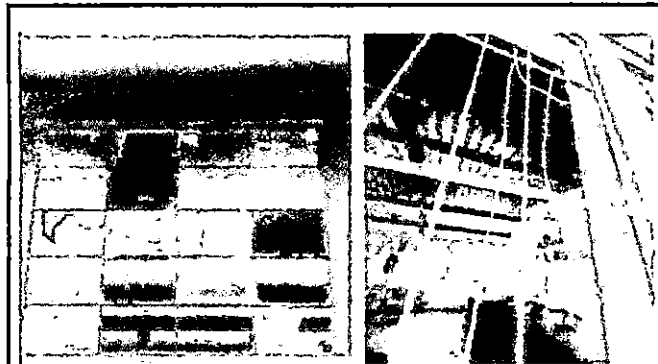
Foto 3: Sustituciones de vidrios, sustitución de balcones de metal, mantenimiento a balcones de metal de 4 aulas.
