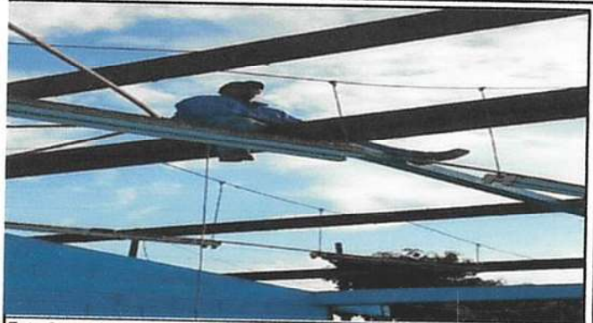
Foto 2: sustitucion de lámina por lamina troquelada aluzin calibre 26
