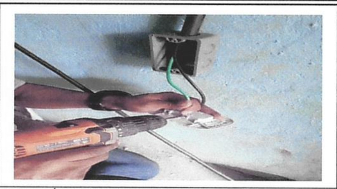
SUSTITUCIÓN DE TOMACORRIENTE DOBLE
