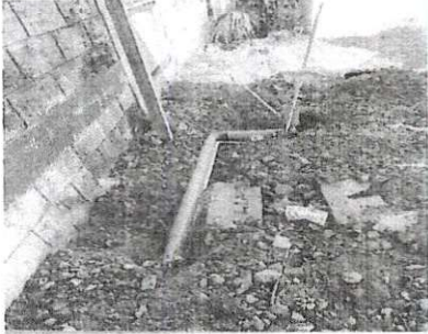
Foto 7: Sustitución de tubería PVC Línea principal aguas negras
