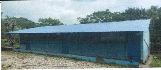
FOTO No. 01 SUSTITUCION DE TECHO DE DURALITA POR LAMINA TROQUELADA
