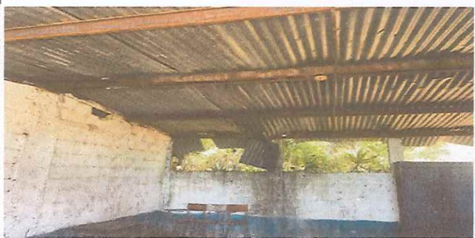
Foto 5: Levantamiento de pared, cambio de estructura metálica y techo. Aula 4
