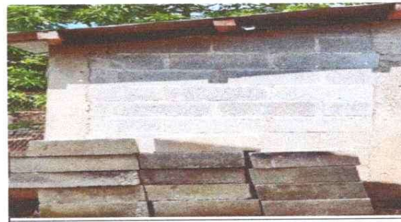
Sustitución de techo de sanitarios, mejoramiento en muro y repello
