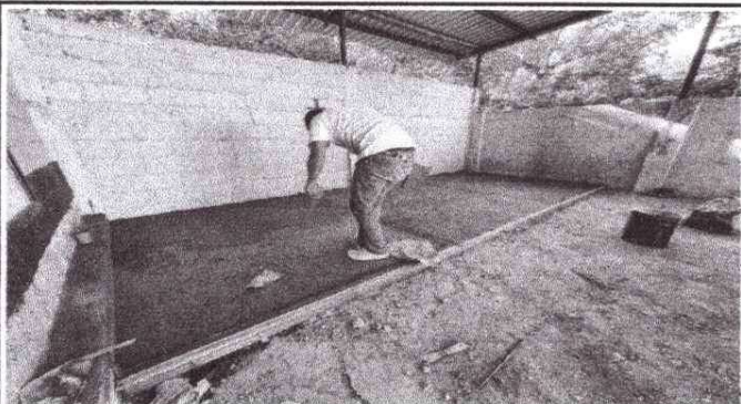
Foto 3: Proceso e instalación de contrapiso.
