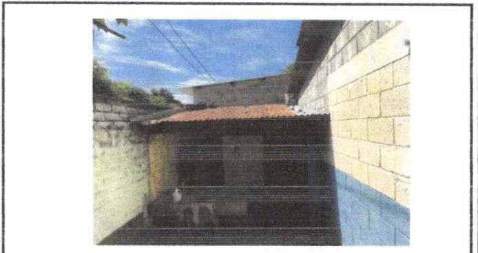
FOTO 4: TECHO EN MAL ESTADO JUNTO CON SU ESTRUCTURA, SE OPTARA POR UN ARREGLO PERMANENTE CON LOSA FUNDIDA DE CONCRETO ARAMADO
