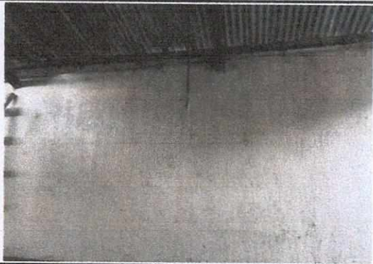
Foto 3: Reforzamiento de pared lateral lado oeste de Cocina con columnas
