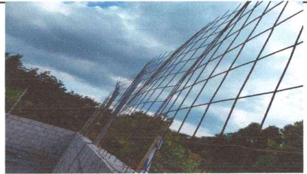
Circulado de Block y Colocación de Electromalla y tubo en la Parte de la Terraza del Establecimiento
