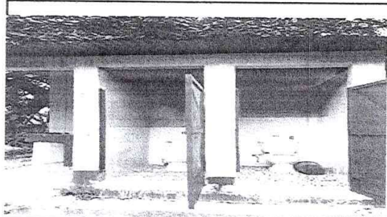
Foto 4: Implemento 1 nuevo sanitario para un total de 2 nuevos y colocó piso y azulejo al fondo se cambio la pila y las mesas de los lavamanos.
