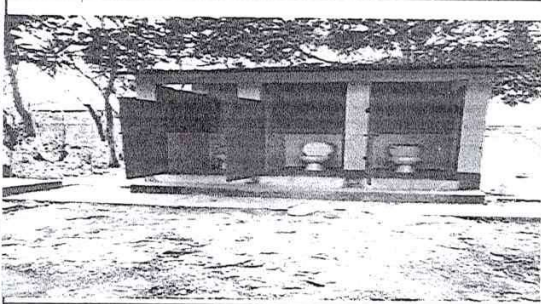
Foto 3: 3 sanitarios de los cuales son nuevos, instaló piso y se colocó azulejo, mesitas para lavamanos.
