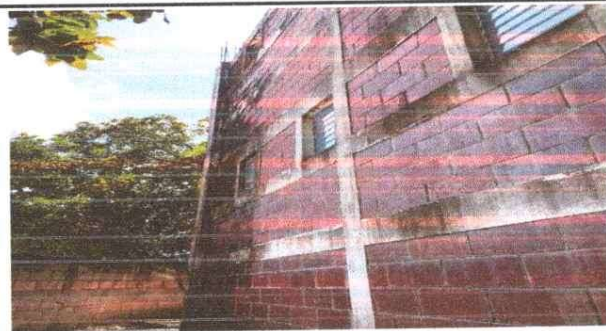
Foto 6: LEVANTAMIENTO DE BORDILLO DE BLOCK REDIRIGIR EL AGUA PLUVIAL HACIA LAS GARGOLAS Y QUE ESTA NO DESCienda POR LA PAREDES
