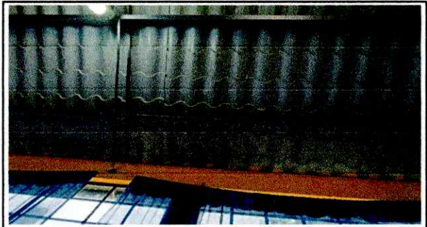
Foto 2: Sustitución de lamina troquelada C24
