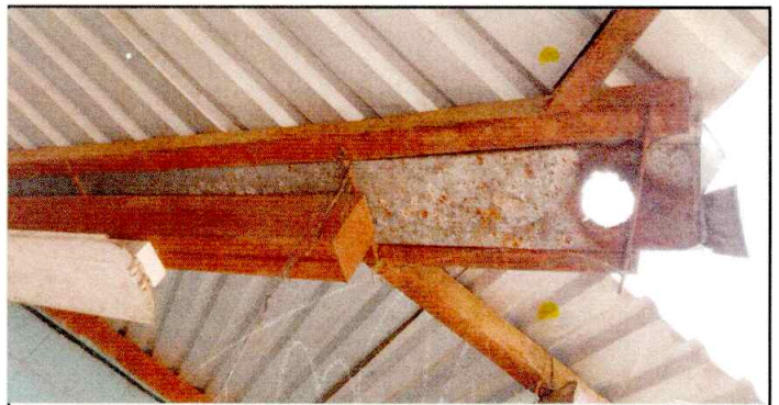
Foto 6: Sustitución de Canal.
