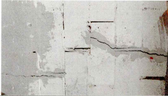
Foto1: Reconstrucción de pared dañada de una aula.
