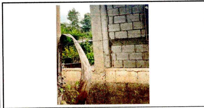
Foto 5: paredes de cocina sin terminar.
