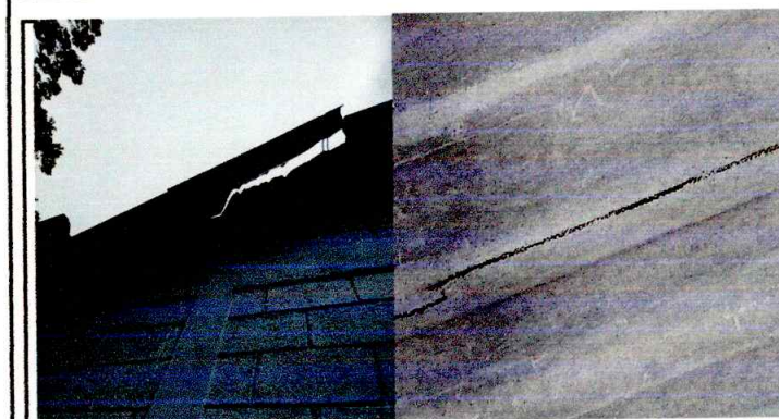
Foto 3: VISTA DE LAS AREAS DONDE SE VE QUEBRADA LA LAMINA DE FIBROCEMENTO INTERNA Y EXTERNA
