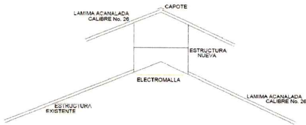
Foto3: DETALLE CONSTRUCTIVO PARA VENTILACION EN LAS AULAS
