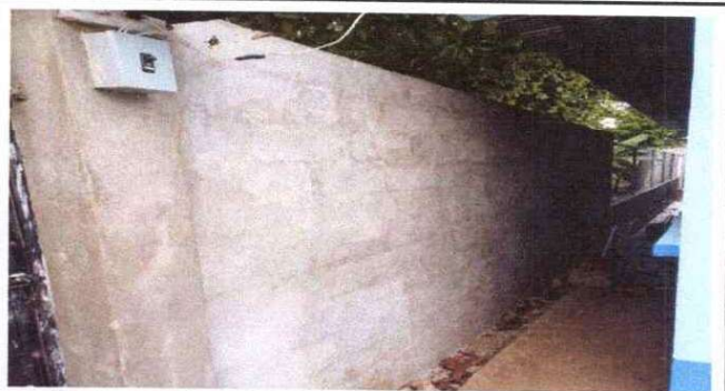
Foto 4: REPARACIÓN DE MURO PERIMETRAL DE BLOCK CON TUBO HG Y MALLA GALVANIZADA SOLERAS Y COLUMNAS PARTE LATERAL DERECHO
