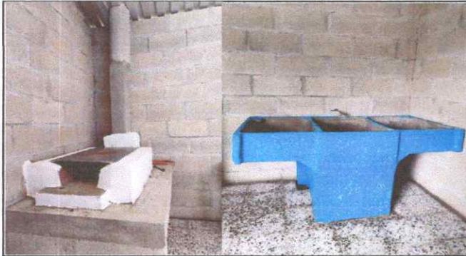
Foto 1: SUSTITUCION DE ESTUFA CON CHIMINEA TERMINADA, PILA DE DOS LAVADEROS TERMINADA
