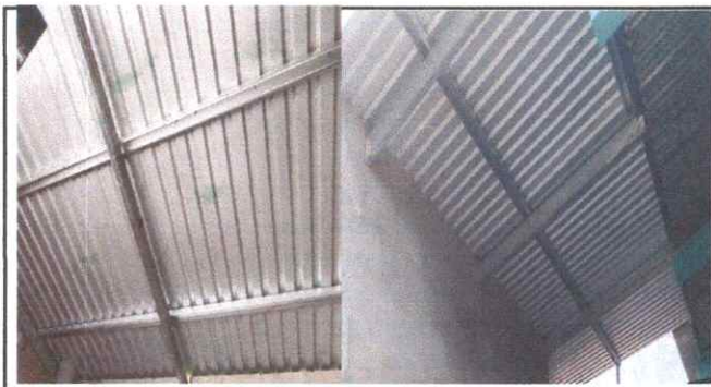
Foto 3: SUSTITUCION DE LAMINA POR LAMINA TROQUELADA TERMINADA. SUSTITUCION DE ESTRUCTURA TERMINADA
