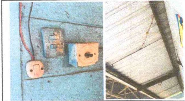
Foto 4: Sustitución de focos ahorradores, sustitución de plafoneras, sustitución de tomacorrientes, cableado electrico y ducto
