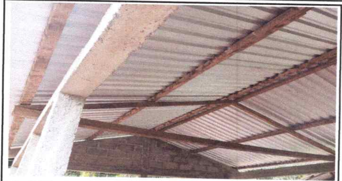
FOTO 2: LEVANTAMIENTO DE ESTRUCTURAS DE MADERA.
