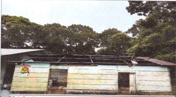
FOTO 1: Sustitucion de lámina, por lámina troquelada Aluzinc calibre 26
