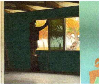
Foto 3: cambio de telas y empaques de las ventanas.
