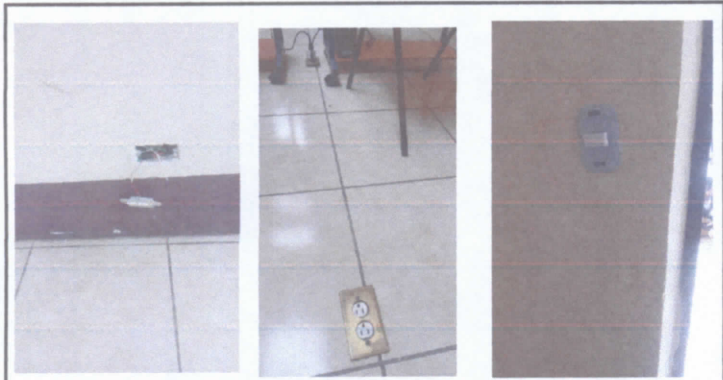
foto No. 24 y 25 sustitución de tomacorrientes dobles. Y foto No. 26 sustitución de interruptores simples y dobles
